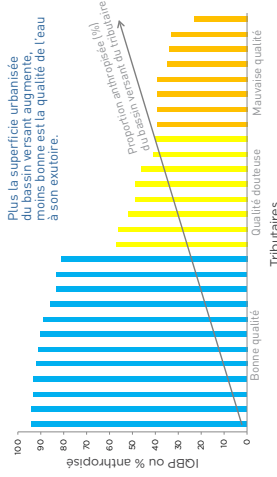
Figure 1. Qualité de l'eau selon l'indice de qualité générale de l'eau du Québec (IGBP 2016) des tributaires du lac Saint-Charles
